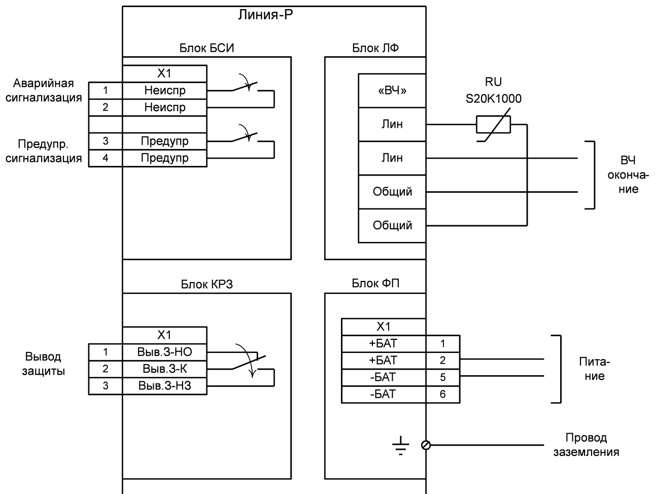
Рисунок 1.1 - Схема подключения цепей питания и ВЧ канала
