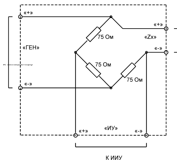
Рисунок 2.8 - Эквивалентная схема измерителя затухания несогласованности PE2.736.000
