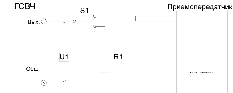
Рисунок 2.6 - Схема измерения уровня порога чувствительности
