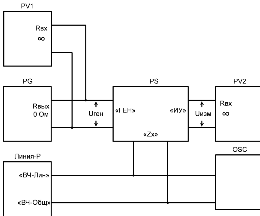
Рисунок 2.7 - Схема проверки затухания несогласованности
